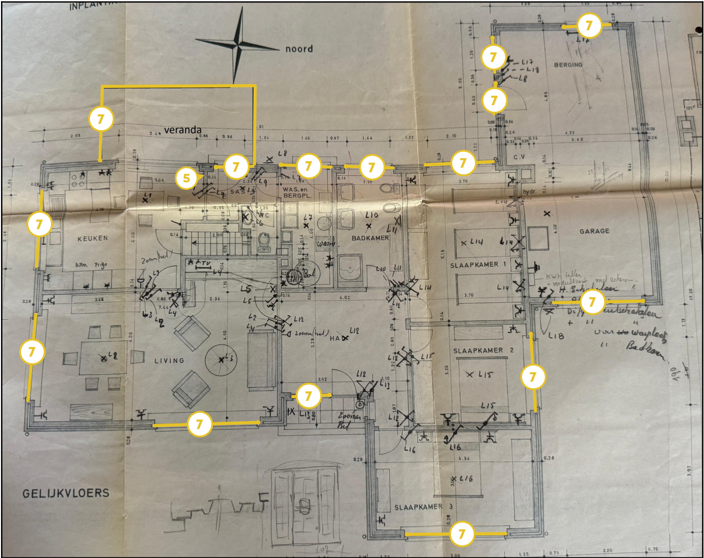
Legende van plan 1.5: Plan gelijkvloers
